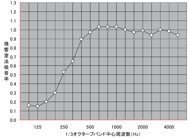
吸音率試験結果
