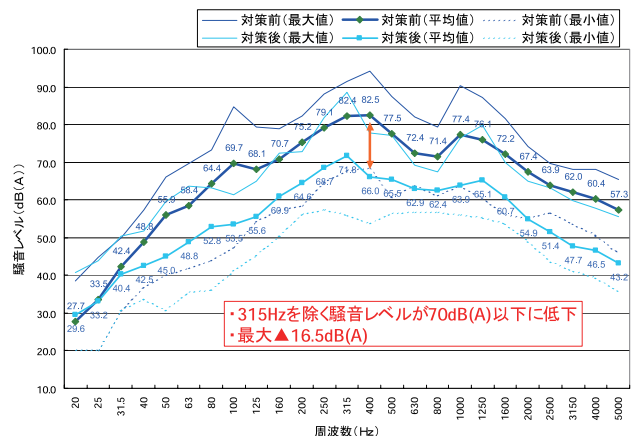
突発騒音 100 台分の周波数分析結果
